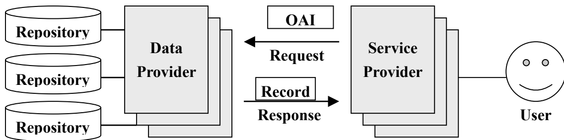
圖一 OAI 結構示意圖
