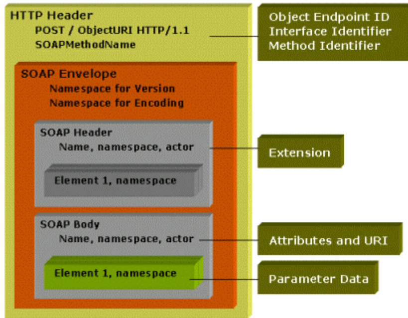
圖二 一個標準的 SOAP 訊息結構 (資料來源：INT Media Group, Incorporated)
